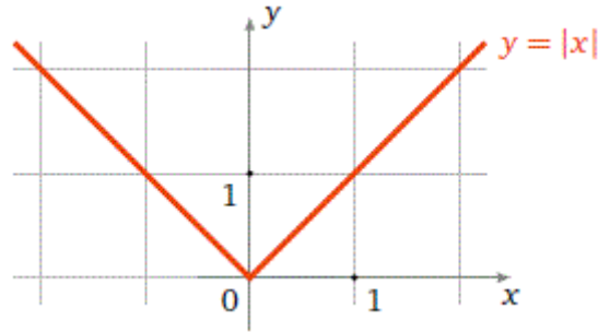
الشَّكْل (5) : تابع القيمة المطلقة
