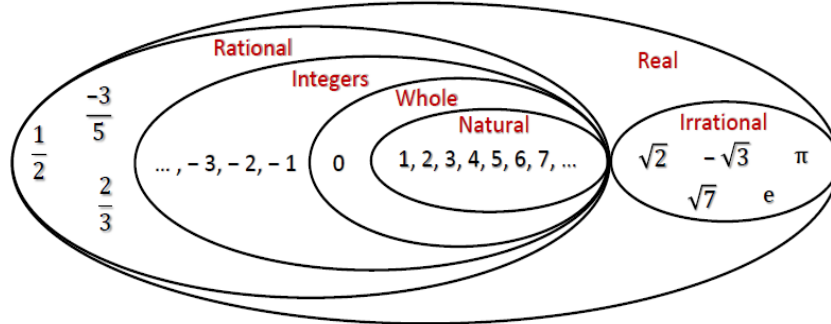
الشكل (3) : المجموعات العددية
