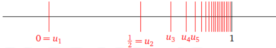
الشكل (9): العنصر الأعظمي والأصغر
