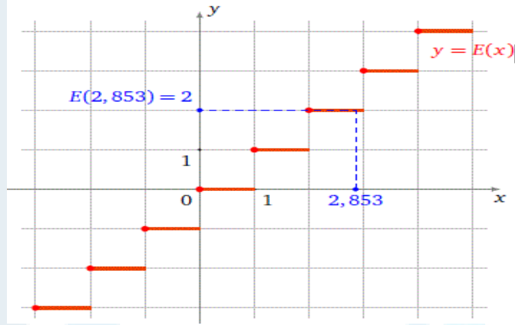
الشّكل (4) : تابع الجزء الصحيح
