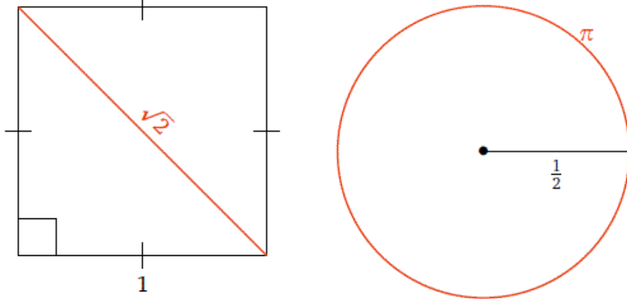
الشكل (1) : ظهور الأعداد غير العاديّة في الأشكال الهندسيّة
