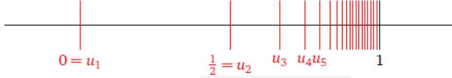
الشكل (9) : العنصر الأعظمي والأصغري
