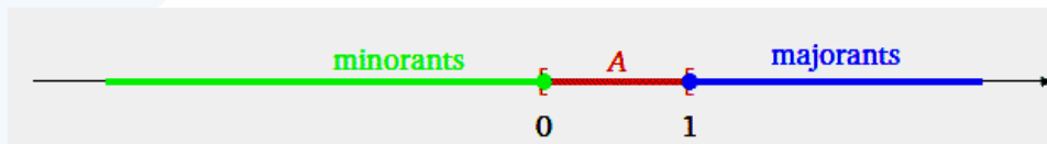
الشكل (10) : الحدود العليا والدنيا لمجموعة
