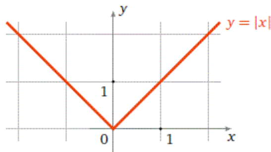
الشكل (5) : تابع القيمة المطلقة
