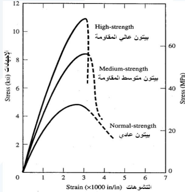
الشكل (4-2): العلاقة ( \sigma - \varepsilon ) لعدة أنواع من البيتون المعرض للضغط البسيط
