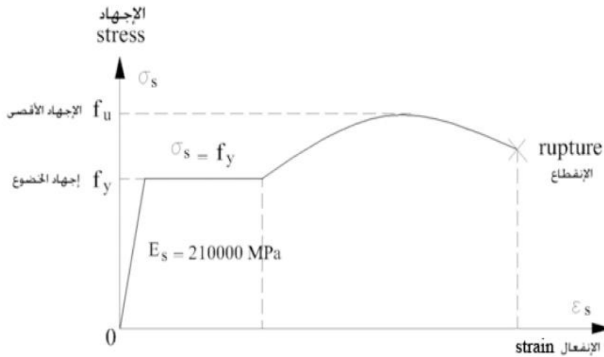
الشكل (10-2): المنحني الافتراضي اجهاد - تشوه (انفعال) للفلود الطري العادي والعالي المقاومة
