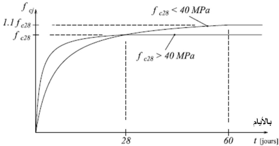
الشكل (5-2): تطور مقاومة الببتون على الضغط البسيط مع الزمن
