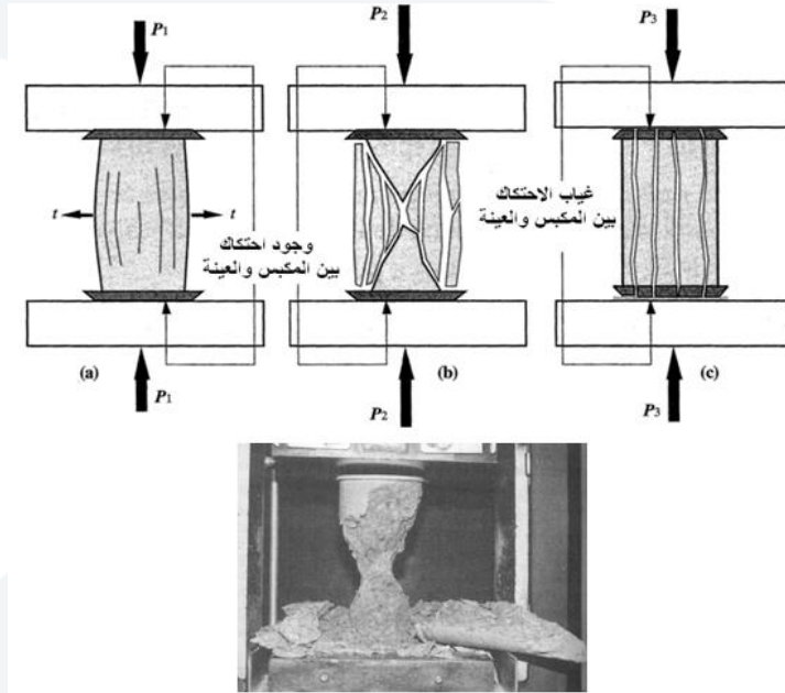
الشكل (2-2): أنماط انهيار عينة بيتونية على الضغط البسيط
