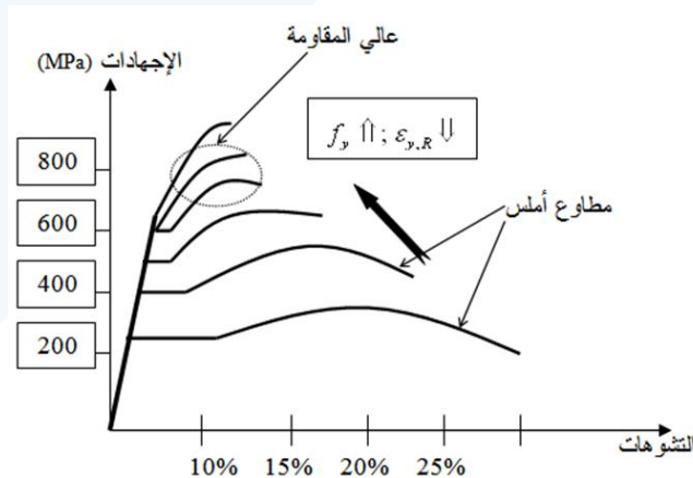
الشكل (9-2): سلوك فولاذ التسليح المطاوع وعالي المقاومة
