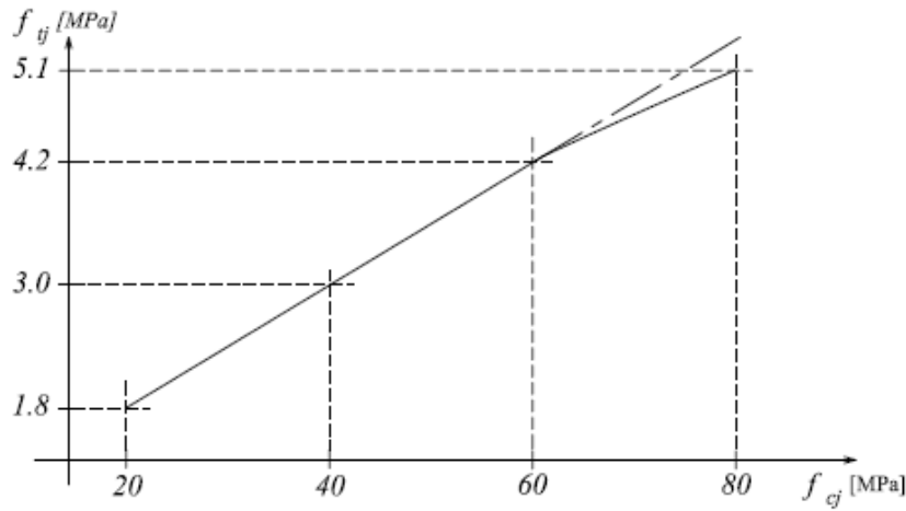
الشكل (6-2): تطور مقاومة البيتون على الشد تبعاً لمقاومته على الضغط البسيط
