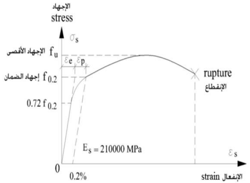
الشكل (2-11): المنحني الافتراضي اجهاد - تشوه (انفعال) للفلوآذ المعالج على البارد
