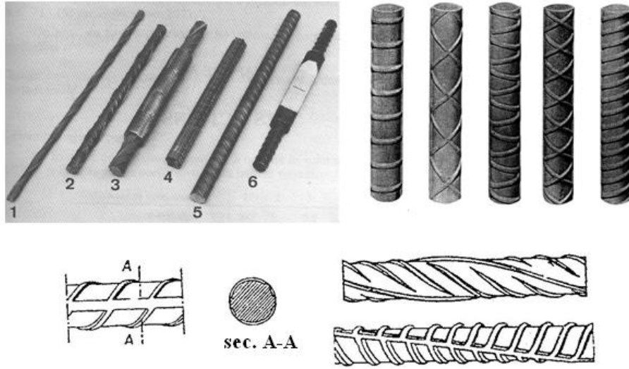
الشكل (7-2): أنواع مختلفة من قضبان التسليح الفولاذية المستخدمة في أعمال البيتون المسلح
