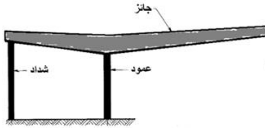
الشكل (6-8): عناصر إنشائية خاضعة لشد بسيط
