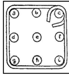
التسليح خارج منطقة الوصل
