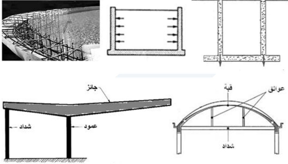
الشكل (6-8): عناصر إنشائية خاضعة لشد بسيط
