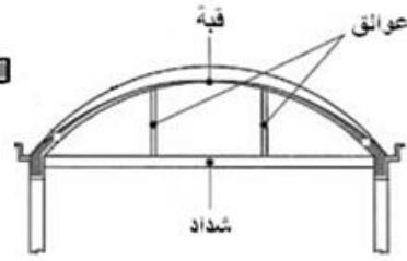
الشكل (6-8): عناصر إنشائية خاضعة لشد بسيط
