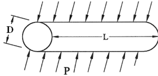
الشكل (8-2): اختبار الشد في البيتون بفلق الأسطوانة
