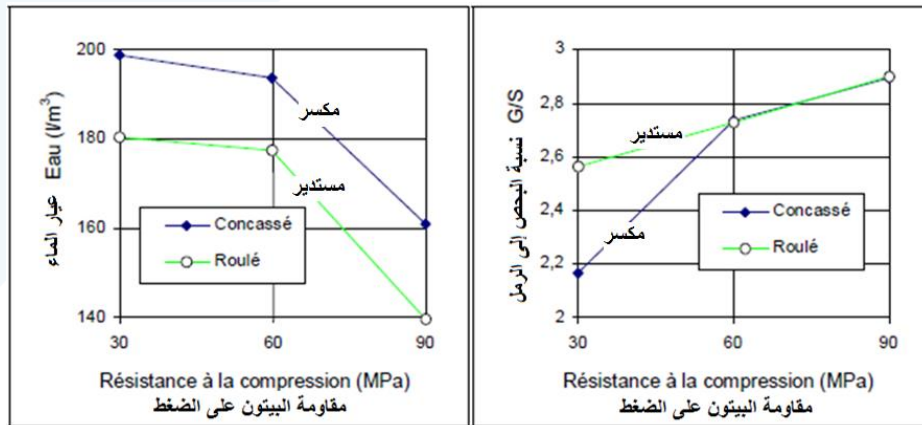
الشكل (4-1): تأثير شكل الحصى على المقاومة
