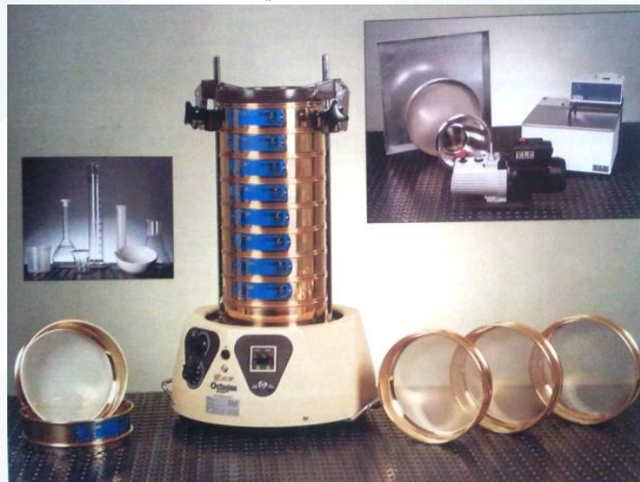
الشكل (7-1): تجربة التحليل الحبي للحصويات الناعمة
