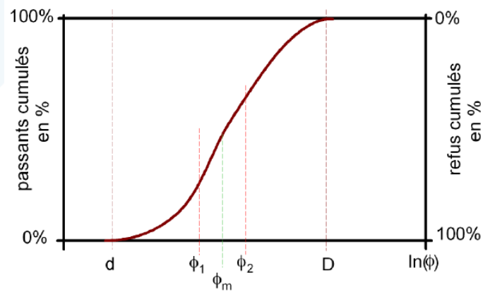
الشكل (7-1): تجربة التحليل الحبي للحصويات الناعمة
