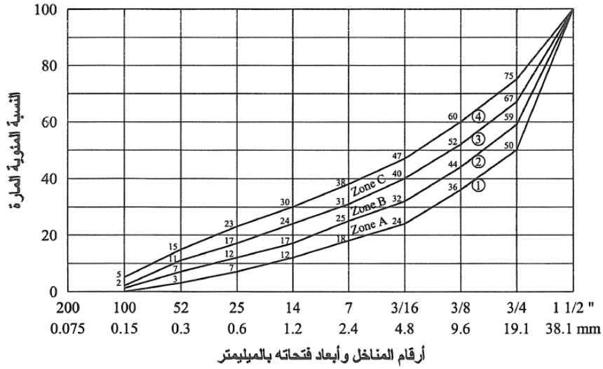
الشكل (12-1): المنحنيات الأربعة للتدرج الحبي للحصويات المكونة للبيتون وفق الكود السوري ( D_{max} = 38 mm )
