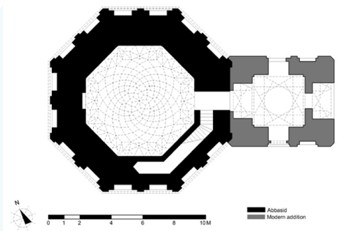
تربة زمرد خاتون في بغداد (الكرخ): المبنى المئمن ذو القبة المخروطية المقرنصة - المسقط
