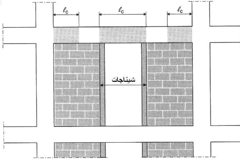
الشكل (5-97): المناطق الحرجة بوجود قواطع
