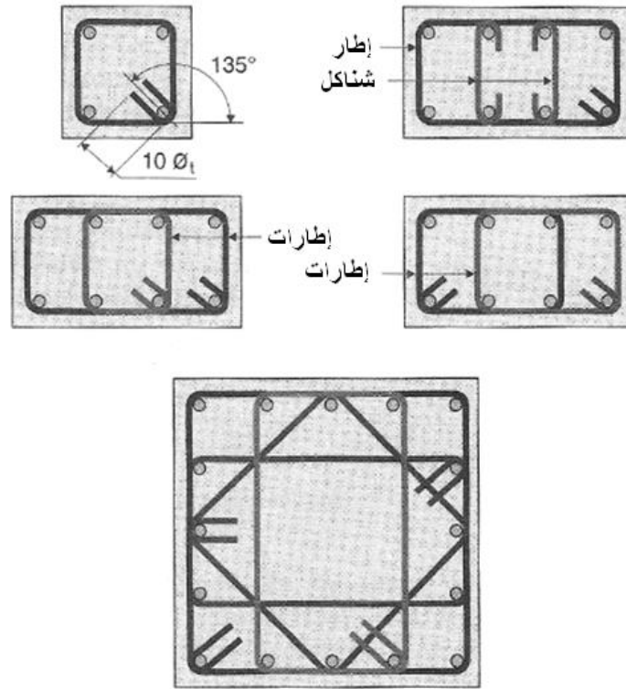
الشكل (5-80): ترتيب وتوضع التسليح العرضي في الأعمدة (ضمان ثبات كل القضبان الطولية)
