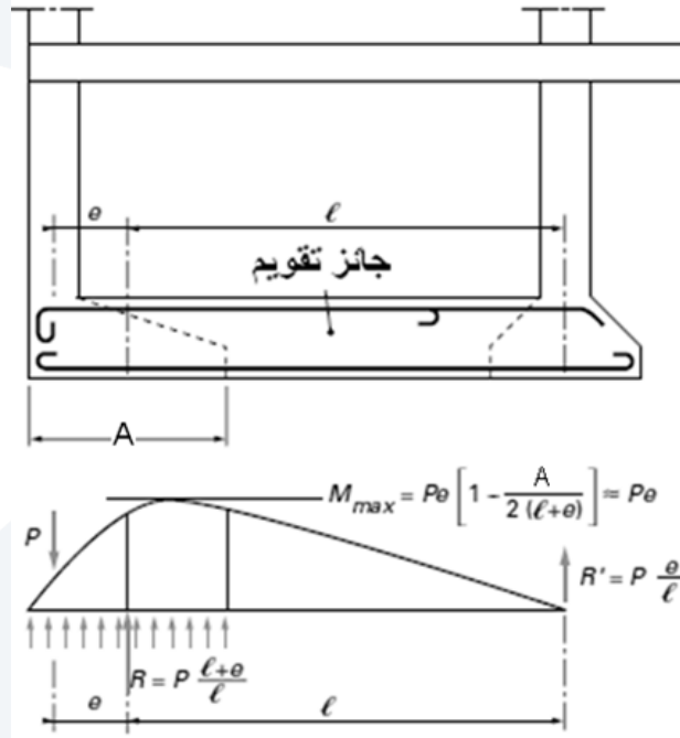
الشكل (5-27): موازنة لامركزية الأساس الطرفي عن طريق جوائز تقويم (مخطط العزم - التسليح)
