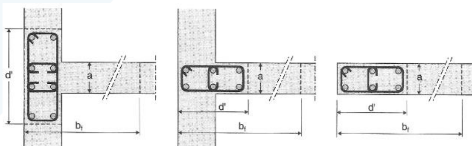
الشكل (5-129): ترتيبات التسليح الطولي لأطراف الجدران المسلحة (أعمدة مخفية)
