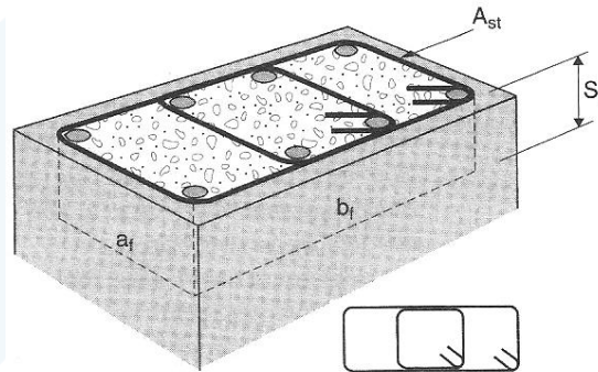
الشكل (5-73): تحديد النسبة الأصغرية للتسليح العرضي (مناطق حرجة)
