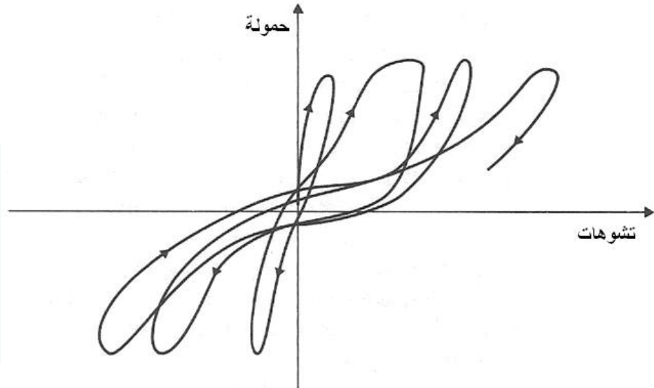
الشكل (6-5): سلوك العناصر الإنشائية تحت تأثير حمولات متناوبة (انتشار التشققات وتدهور التلاحم)
