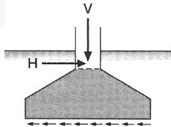
الشكل (10-5): تأمين الاستقرار بالاحتكاك لأساس عادي
