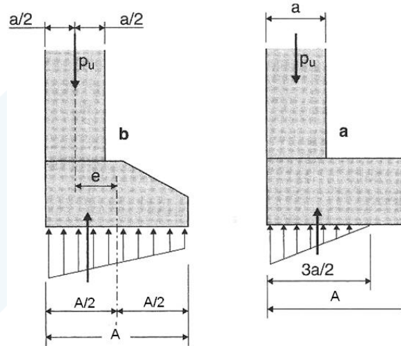
الشكل (5-23): موازنة اللامركزية بالتربة (اجهادات مثلث وشبه منحرف)
