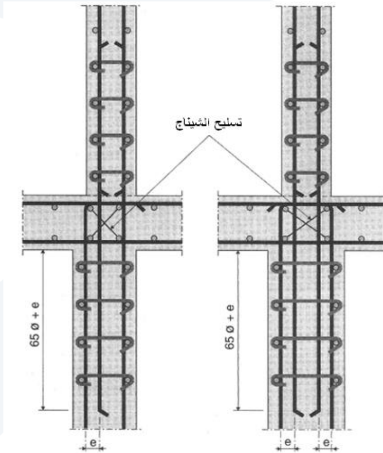
الشكل (5-134): الوصل في حال تغير سماكة الجدار
