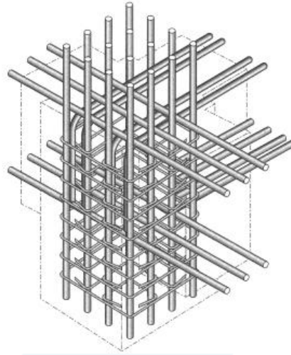
الشكل (5-116): تسليح عقدة جانبية
