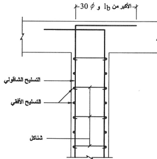
الشكل (5-141): تسليح الجدران الحاملة
