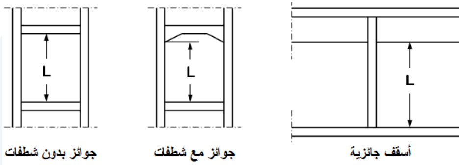
الشكل (52-5): الطول الحر للأعمدة ( L )
