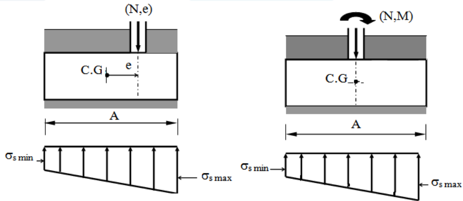
الشكل (5-20): توزيع ضغط التربة تحت الأساس الصلب (حمولة لامركزية)
