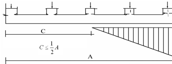
الشكل (5-40): أساس خطي من البيتون المسلح
