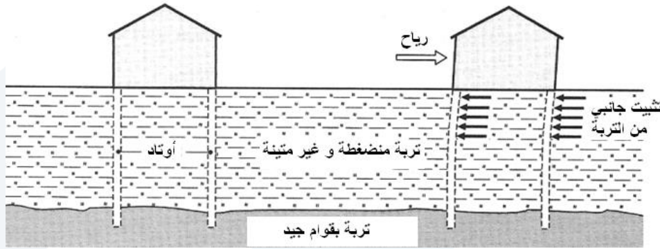
الشكل (5-15): نقل الجهود الأفقية إلى التربة عن طريق الأوتاد (من فعل الرياح)
