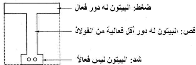
الشكل (5-94): مفاهيم التصميم للعناصر المنعطفة
