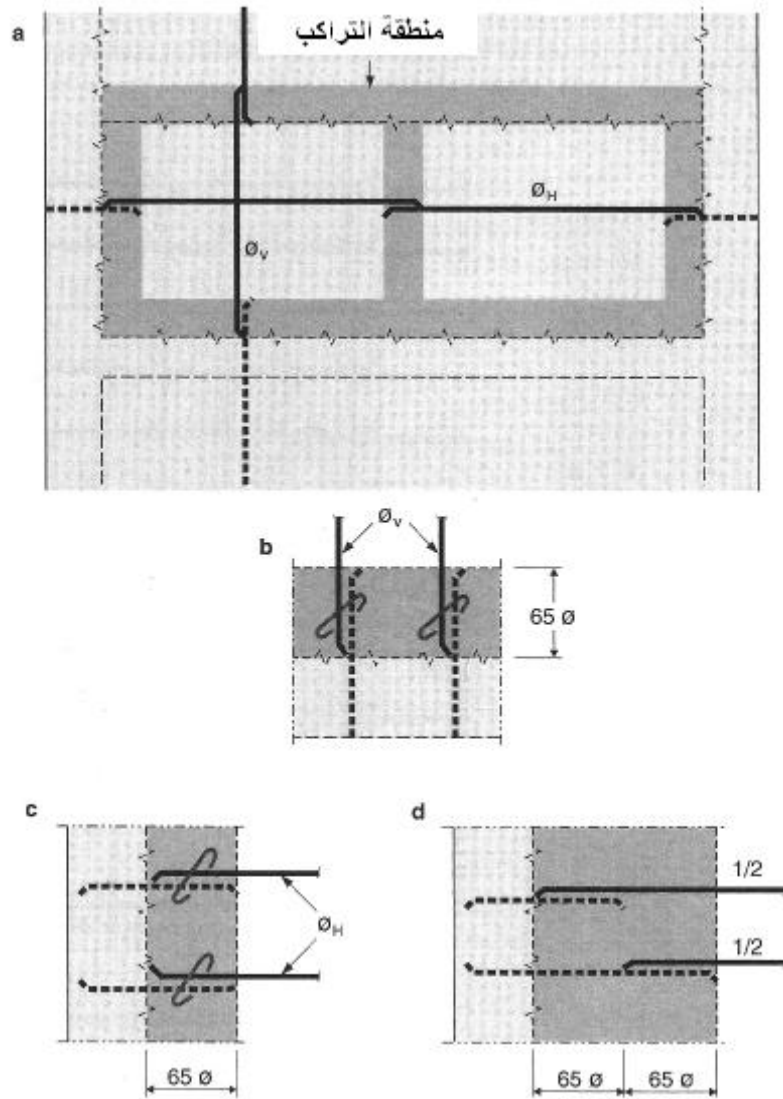
الشكل (5-133): توضع الشناكل في مناطق التراكب
