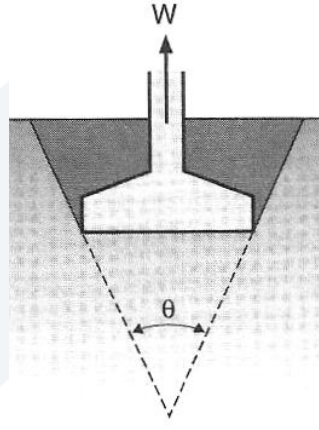
الشكل (12-5): مقاومة الرفع بموشور تربة زاويته \theta = 60^\circ
