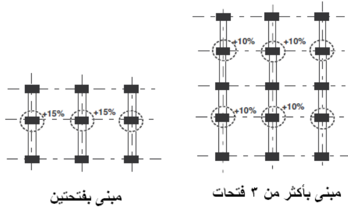
الشكل (5-55): زيادة الحمولات الطابقية للأعمدة
