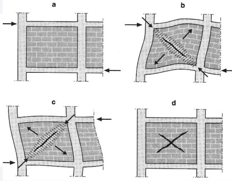
الشكل (5-118): عمل جدار الملى الخاضع لقوى أفقية
