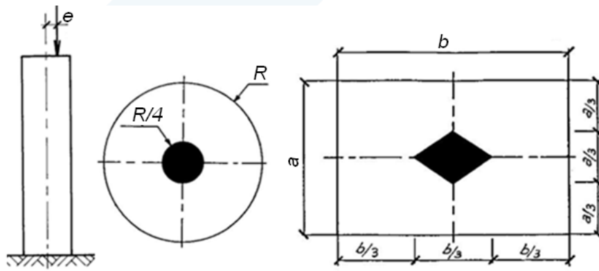
الشكل (44-5): النواة المركزية لمقطع مستطيل ودائري
