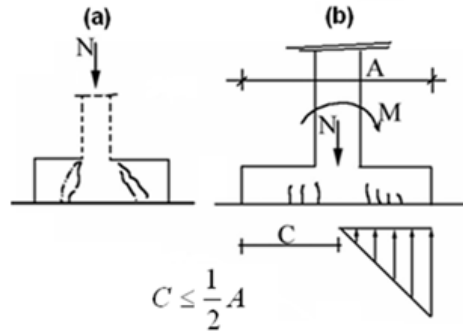
(a) أساس منفرد من البيتون غير المسلح، (b) أساس منفرد من البيتون المسلح، الشكل (41-5): التشيقات في أساس سطحي منفرد
