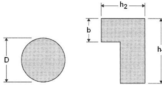
الشكل (5-66): الأبعاد الأصغرية للأعمدة
