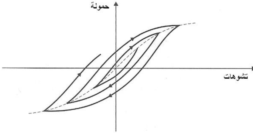
الشكل (5-5): سلوك العناصر الإنشائية تحت تأثير حمولات متناوبة (حالة عدم تأثر الصلابة والمقاومة)
