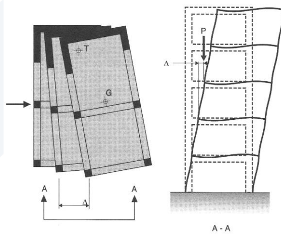
الشكل (5-74): تشوهات الأعمدة الركنية في حالة الفتل حول محور شاقولي
