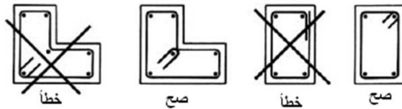
الشكل (5-82): نماذج من التسليح العرضي الواجب تجنبه
