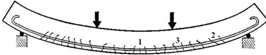
الشكل (5-93): التشققات في جانز محمل - تطور جهة التضررات
