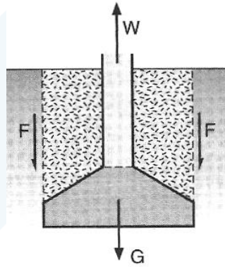
الشكل (13-5): مقاومة الرفع بموشور تربة قائم
