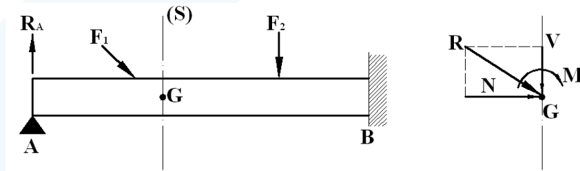
الشكل (57-5): عنصر إنشائي خاضع لانعطاف مركب
