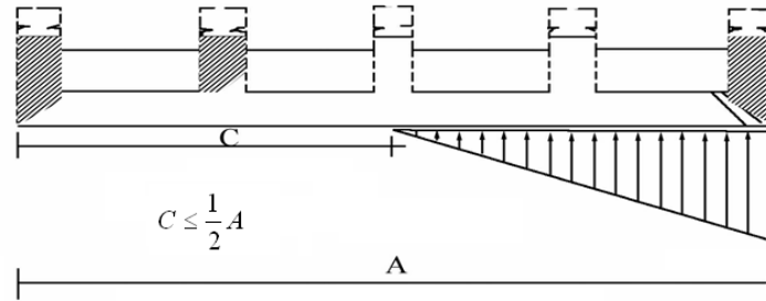
الشكل (5-39): أساس حصيرة من البيتون المسلح
