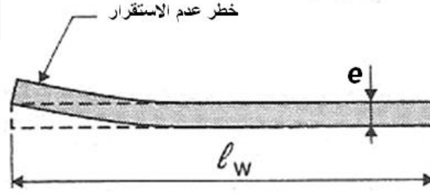
الشكل (5-123): عدم استقرار جانبي للجدران
