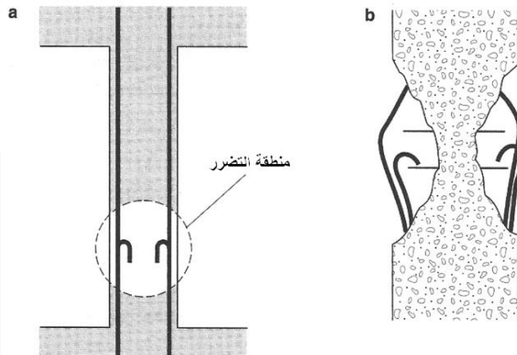
الشكل (5-79): تضرر البيتون في حال وجود عكفات للتسليح الطولي (يمنع استخدام العكفات)
