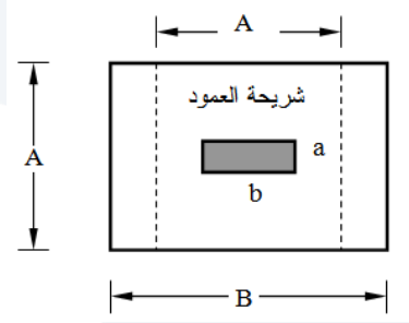
الشكل (35-5): شريحة عمود مستطيل
