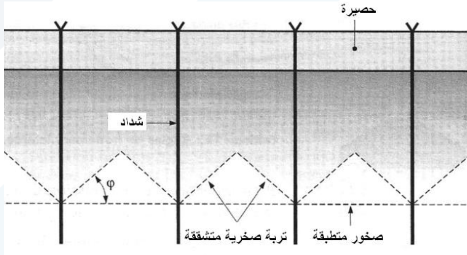
الشكل (5-14): مقاومة الرفع بواسطة زرع شدادات في التربة
