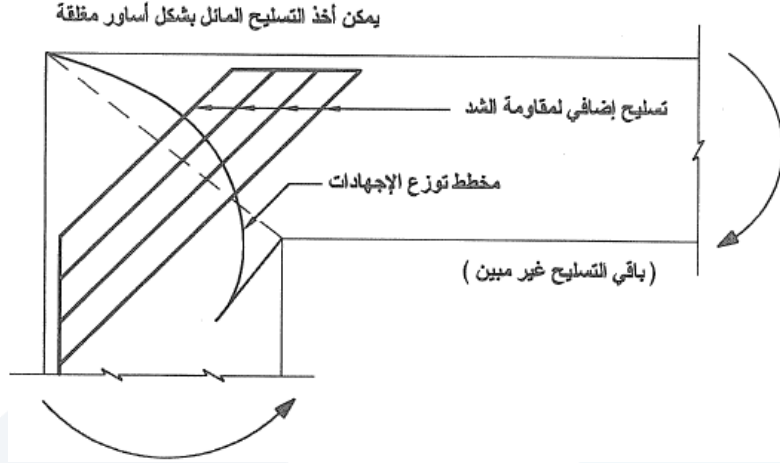
الشكل (5-104): إضافة تسليح خاص في عقدة طرفية لإطار مجازه يزيد عن عشرة أمتار
