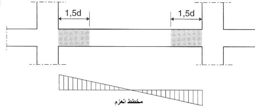
الشكل (5-95): المناطق الحرجة في جوائز ما
