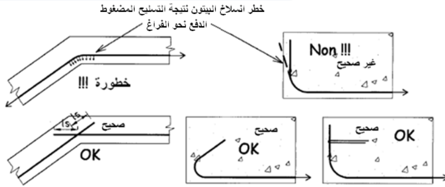
الشكل (5-110): إرساء التسليح الطولي في الجوائز
