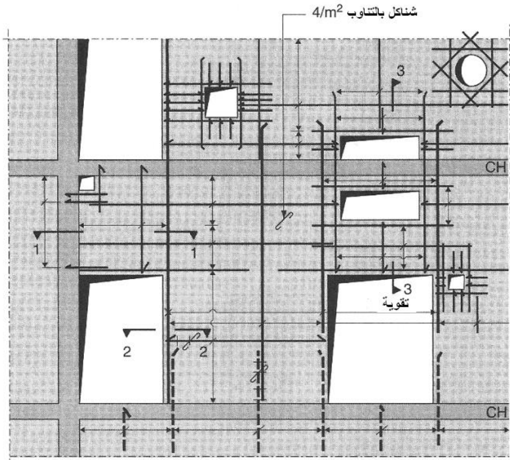
الشكل (5-136): مثال على تسليح جدار (حالة عامة)
