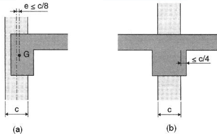
الشكل (5-67): الموقع النسبي للجوائز والأعمدة
