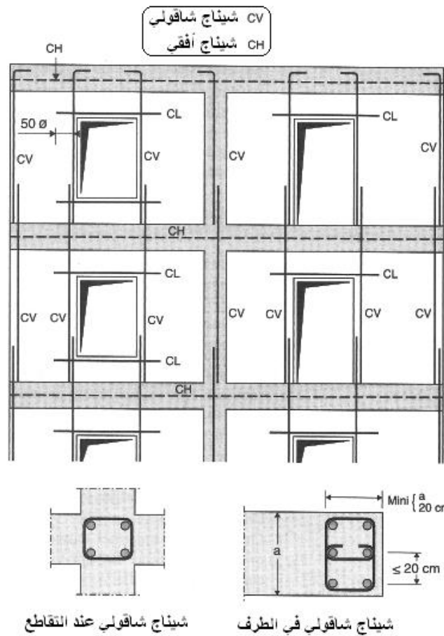
الشكل (5-128): ترتيبات التسليح الأصغري لأطراف الجدران غير المسلحة (الشيناچات)
