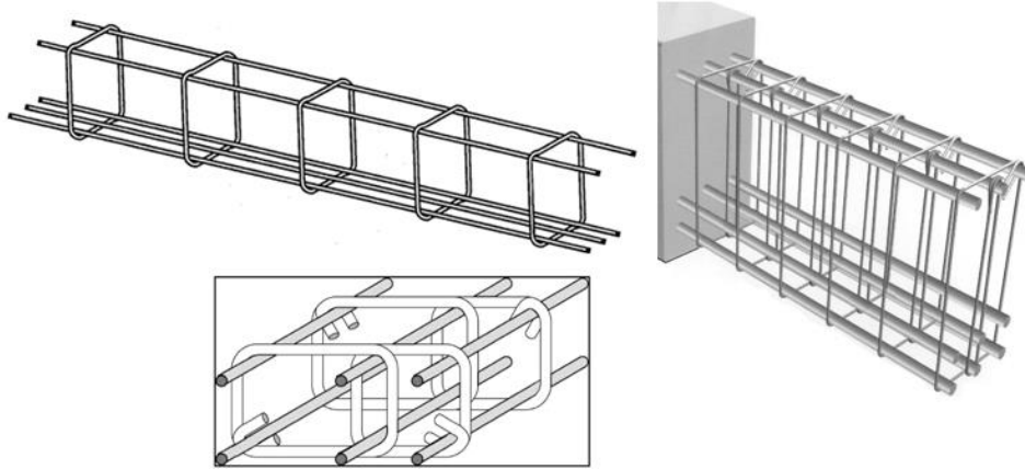
الشكل (5-106): التسليح الطولي والعرضي في الجوائز
