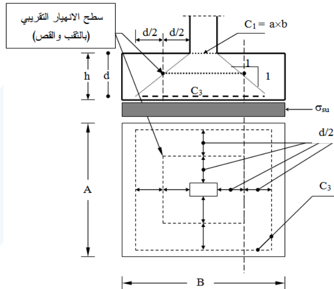
الشكل (5-34): سطوح الانهيار بالثقب والقص
