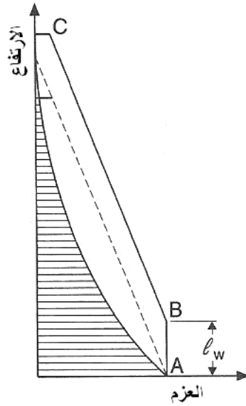
الشكل (5-125): مغلف العزم التصميمي لجدار قص
