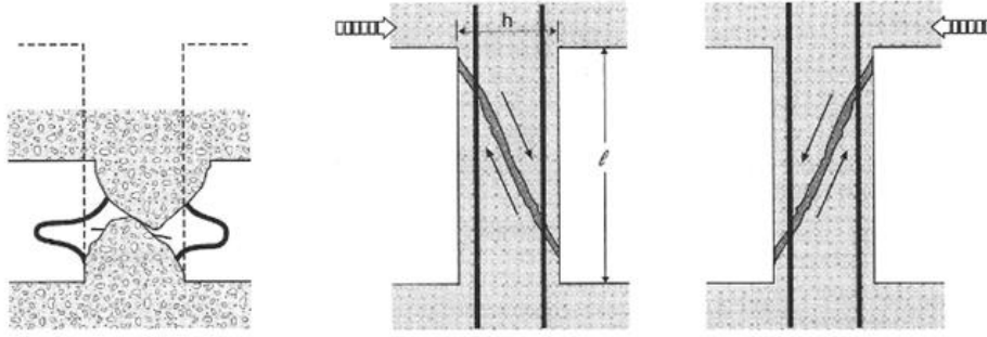
الشكل (76-5): ميكانيزم تضرر الأعمدة القصيرة
