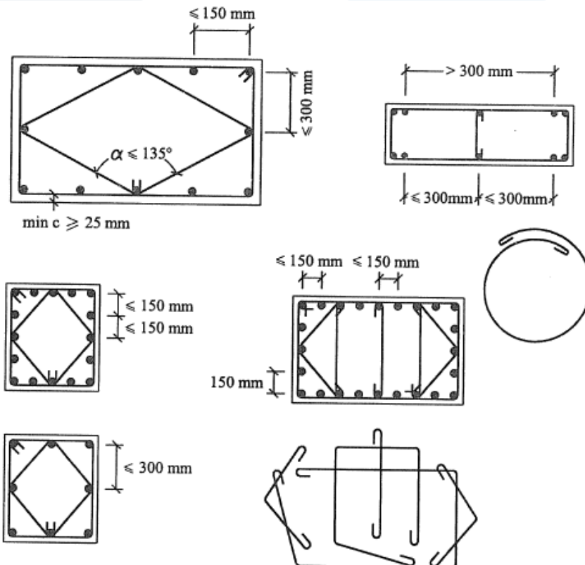
الشكل (5-84): ترتيبات التسليح في الأعمدة (الكود السوري)
