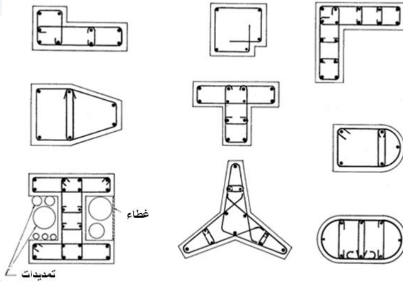
تابع للشكل (5-83): نماذج تسليح مقاطع الأعمدة بأشكال مختلفة
