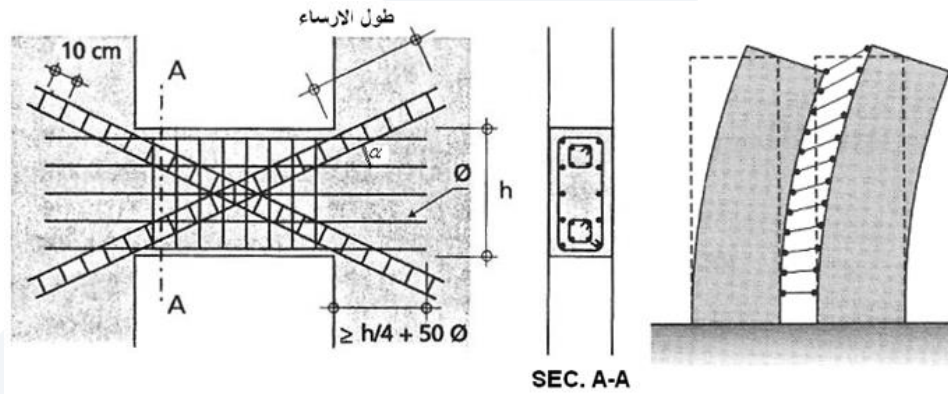
الشكل (5-126): تشكل مفاصل لدنة في اللمعات
