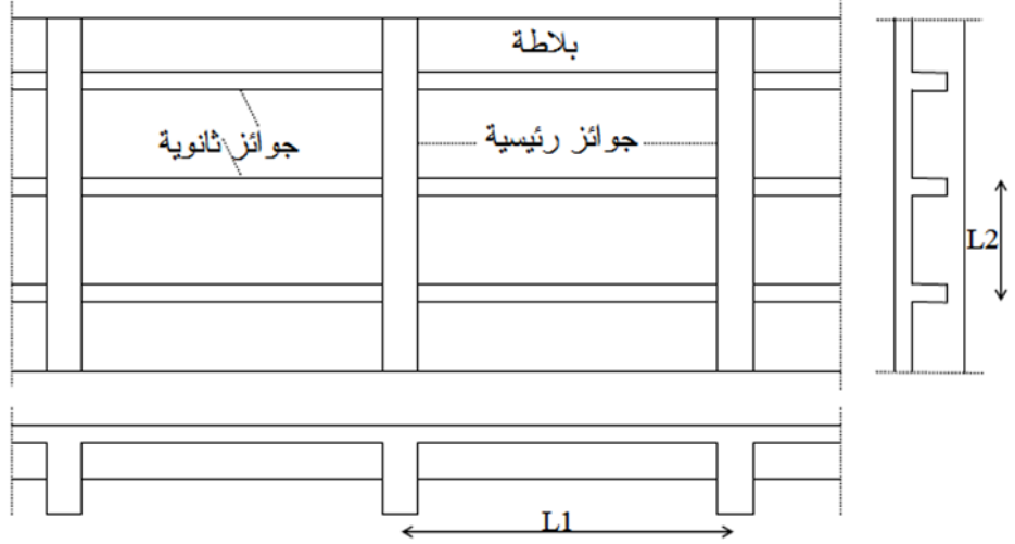
الشكل (5-85): بلاطة سقف مع الجوائز
