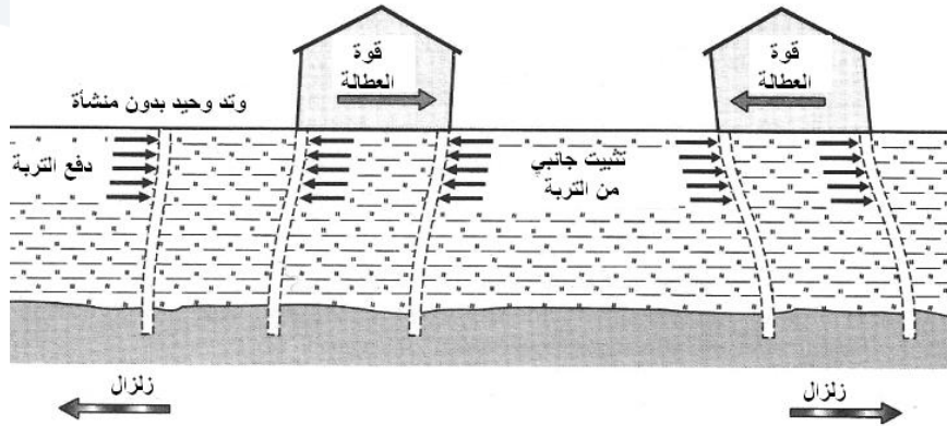
الشكل (5-16): نقل الجهود الأفقية إلى التربة عن طريق الأوتاد (من فعل الزلازل دون معول أو تثبيت جانبي من منشأة تحتية)
