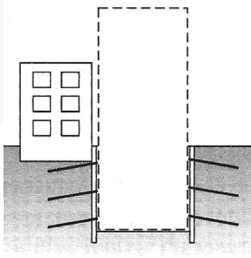
الشكل (5-1): التأسيس وتأمين الحفرة بجوار مبنى قائم
