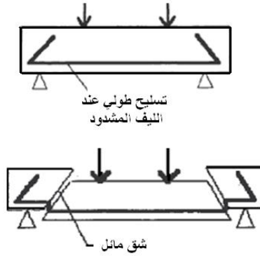
الشكل (5-88): انهيار جائر بيتوني بسبب عدم كفاية البيتون لمقاومة القص
