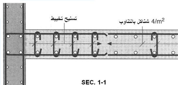
تابع للشكل (5-136): مقطع 1-1
