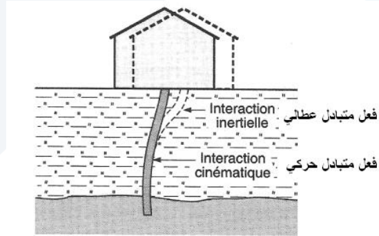
الشكل (5-17): نقل الجهود الأفقية إلى التربة عن طريق الأوتاد (من فعل الزلازل: فعل متبادل حركي وعطالي)
