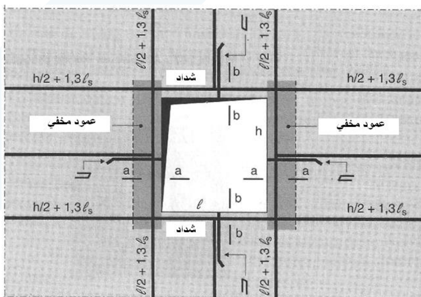
الشكل (5-134): الوصل في حال تغير سماكة الجدار
