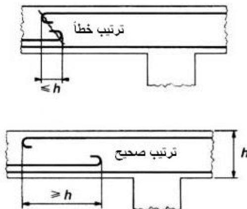
الشكل (5-112): التباعد بين قضبان التسليح الموقوفة (سفلي وعلوي)
