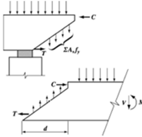
الشكل (5-92): مخطط الجسم الحر في طرف الجانز
