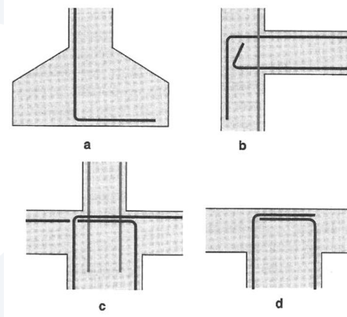
الشكل (9-5): إرساء القضبان بعكفات مستقيمة نظامية
