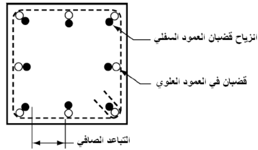
الشكل (5-78): ترتيب وتوضع التسليح الطولي في الأعمدة
