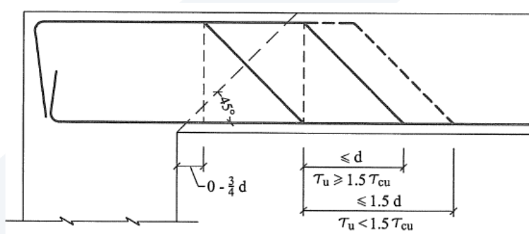
الشكل (103-5): ترتيب القضبان الطولية المكسحة عند المسند
