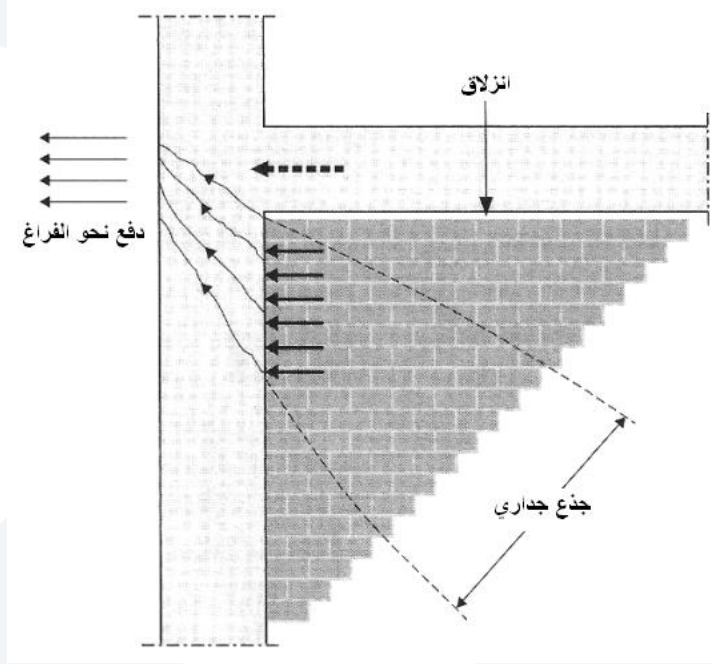
الشكل (5-119): توازن الجهود في حال وجود فاصل غير مملوء بين الجدار والجائز
