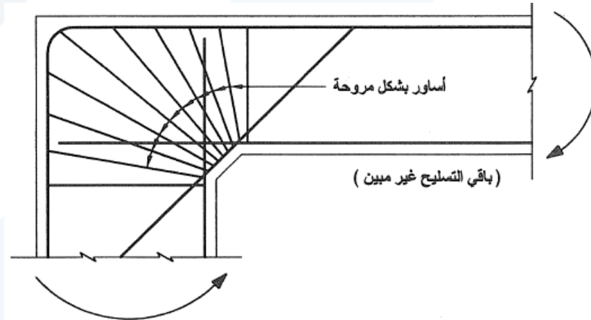
الشكل (5-105): استمرار أساور العمود ضمن العتد، أو تزويدها بأساور بشكل مروحة
