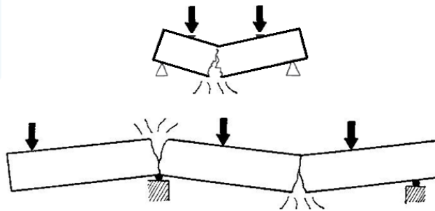
الشكل (5-87): انهيار جانز بيتوني غير مسلح عند مناطق الشد القصوى
