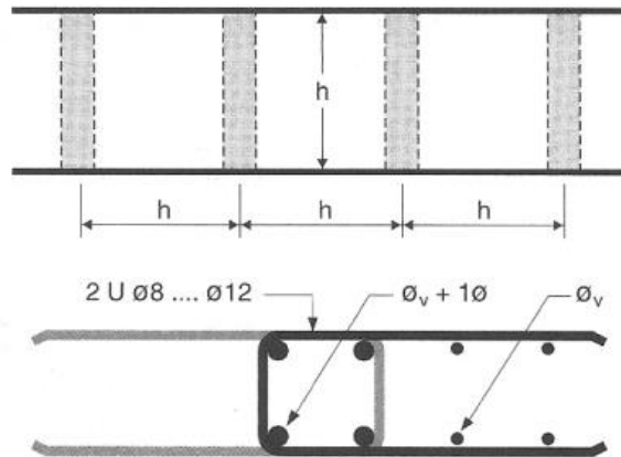
الشكل (5-137): شيناجات شاقولية إضافية بتباعد يساوي ارتفاع الطابق
