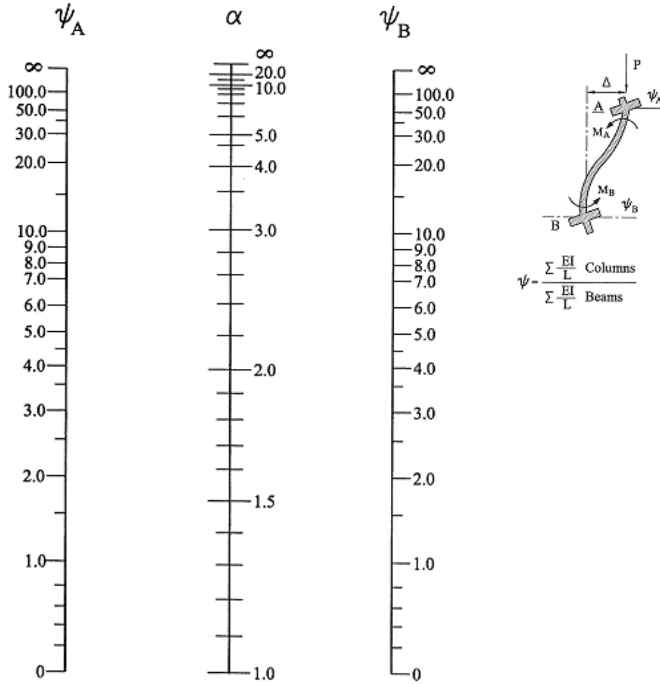
الشكل (53-5): تحديد قيمة \alpha تبعاً لقيمة \Psi_{A,B}
