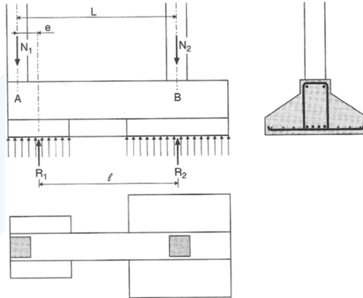
الشكل (5-28): موازنة الحمولات اللامركزية في الأعمدة عن طريق مزدوجة ردود الأفعال بالأساسات
