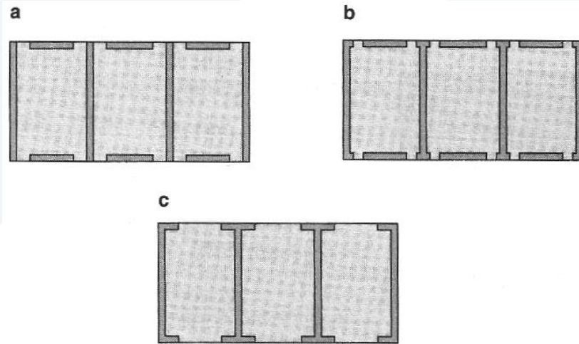
الشكل (5-124): تقوية أطراف الجدران
