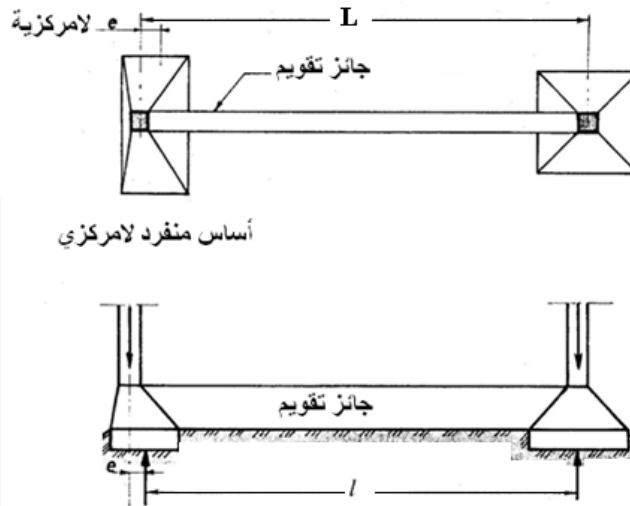
الشكل (5-26): استخدام جائز تقويم صلب يصل بين أساس طرقي و داخلي مجاور
