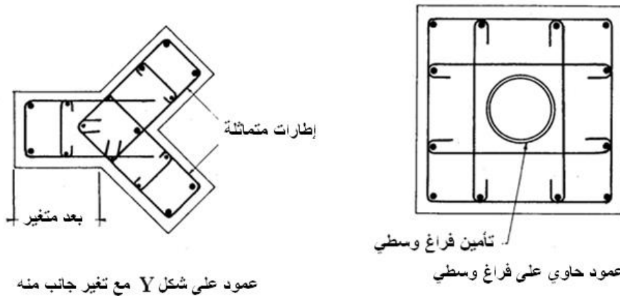
الشكل (5-83): نماذج تسليح مقاطع الأعمدة بأشكال مختلفة
