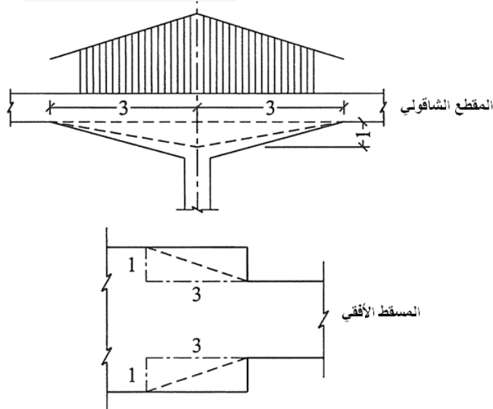
الشكل (5-102): تغير المقاطع عند المساند
