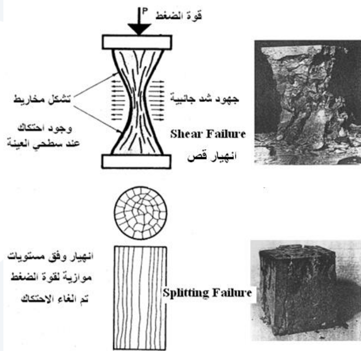
الشكل (5-47): أنماط انهيار عينة بيتونية على الضغط المركزي
