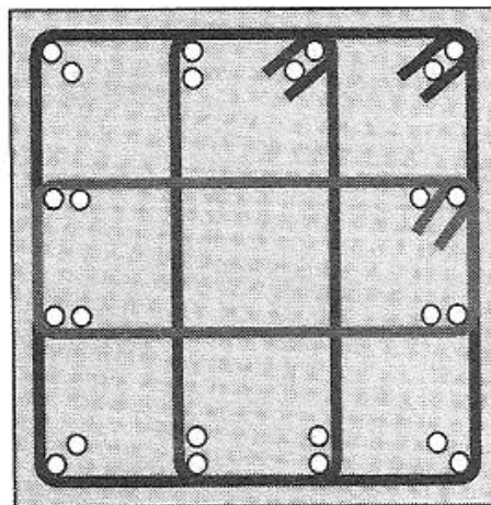
الشكل (5-81): التسليح العرضي في حال استخدام رزم قضبان طولية (يفضل تجنب استخدام الرزم)
