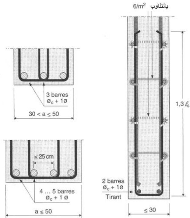
تابع للشكل (5-135): المقطع b-b - تقوية أفقية
