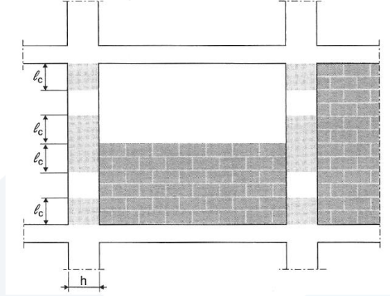
الشكل (5-71): المناطق الحرجة في حالة القواطع غير الكاملة
