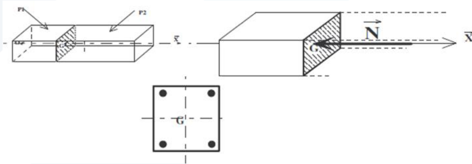
الشكل (42-5): مقطع معرض للضغط البسيط
