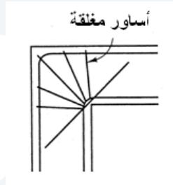
الشكل (5-64): تفصيلاً عقدة معرضة لعزوم متناوبة
