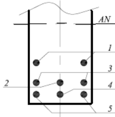
الشكل (5-111): تسلسل إيقاف قضبان التسليح في مقطع الجائز
