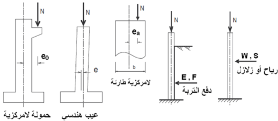
الشكل (43-5): عدم تطابق بين مركز مرور القوة الخارجية ومركز ثقل العمود (لا مركزية)
