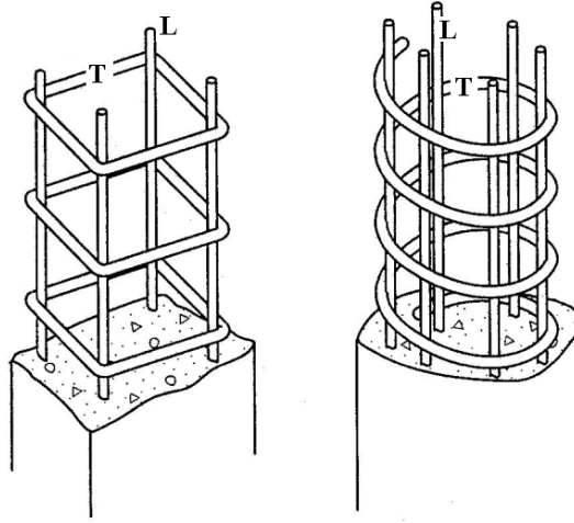
الشكل (45-5): أنواع التسليح في الأعمدة (طولي وعرضي: L & T)
