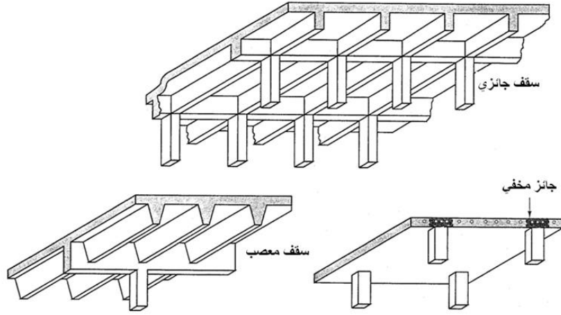
الشكل (5-86): منظومة البلاطات والأعمدة
