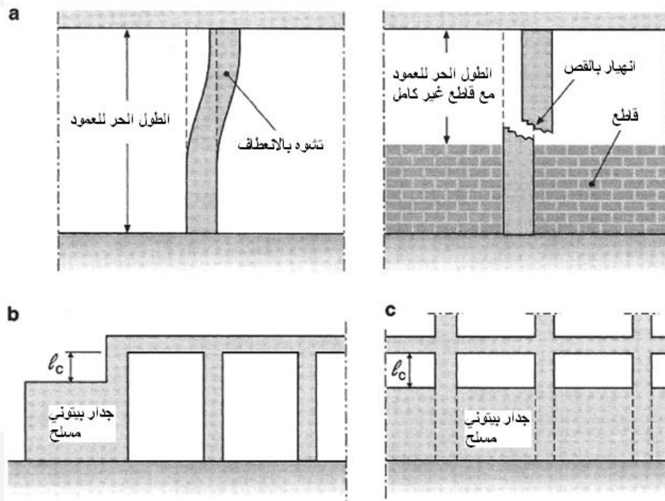
الشكل (5-77): منشآت حاوية على أعمدة قصيرة
