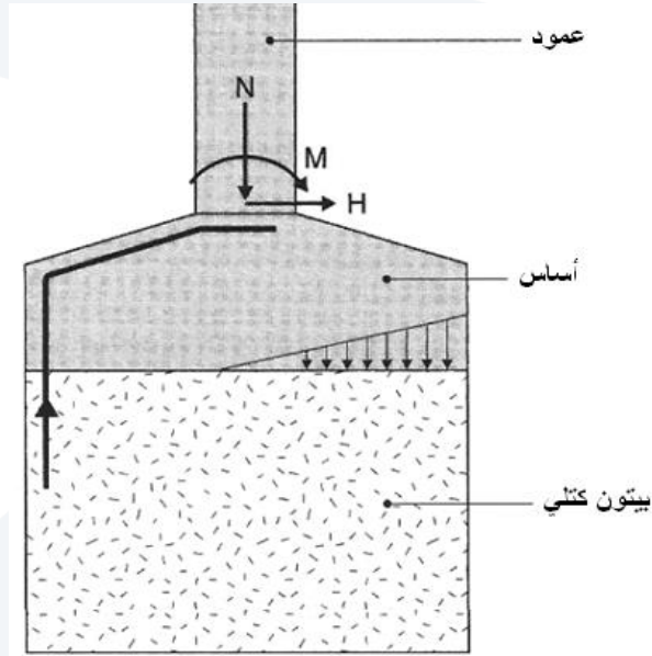
الشكل (5-38): مقاومة قوى الشد عن طريق إرساء التسليح في البيتون الكتلي (تسليح ربط)
