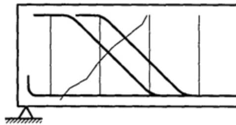
الشكل (5-89): إضافة تسليح عرضي (أساور أو مكسح) لمقاومة القص
