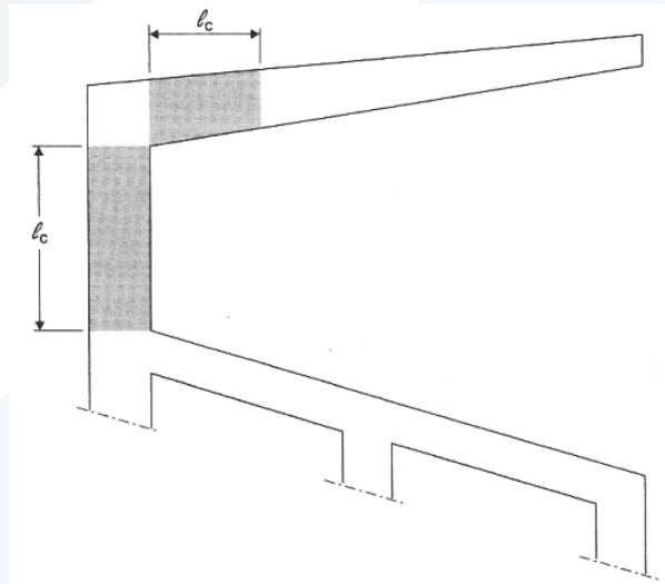
الشكل (5-70): المناطق الحرجة لعمود في ملعب رياضي (ستاد)
