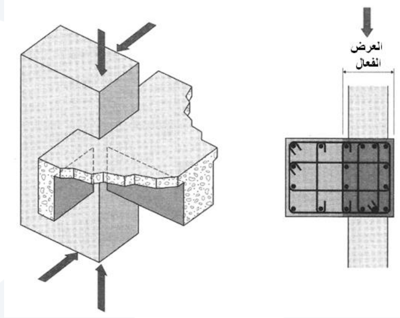
الشكل (5-68): العرض الفعال للعمود عندما يكون e > c/8
