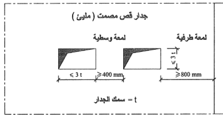
الشكل (5-143): اشتراطات أبعاد الفتحات واللمعات في جدران القص
