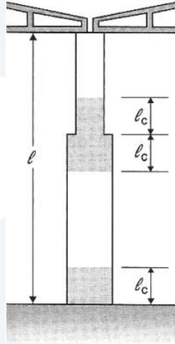
الشكل (5-72): المناطق الحرجة في عمود حامل لسكة رافعة
