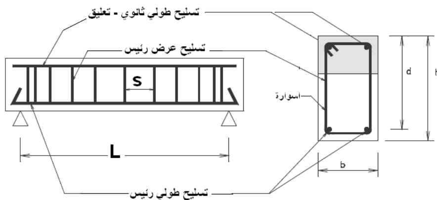
الشكل (5-90): جائر بيتوني مسلح لمقاومة الانعطاف والقص
