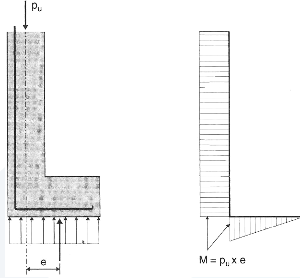
الشكل (5-24): موازنة اللامركزية بالجدار
