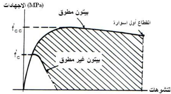
الشكل (5-48): تأثير التطويق على سلوك البتون المعرض لضغط
