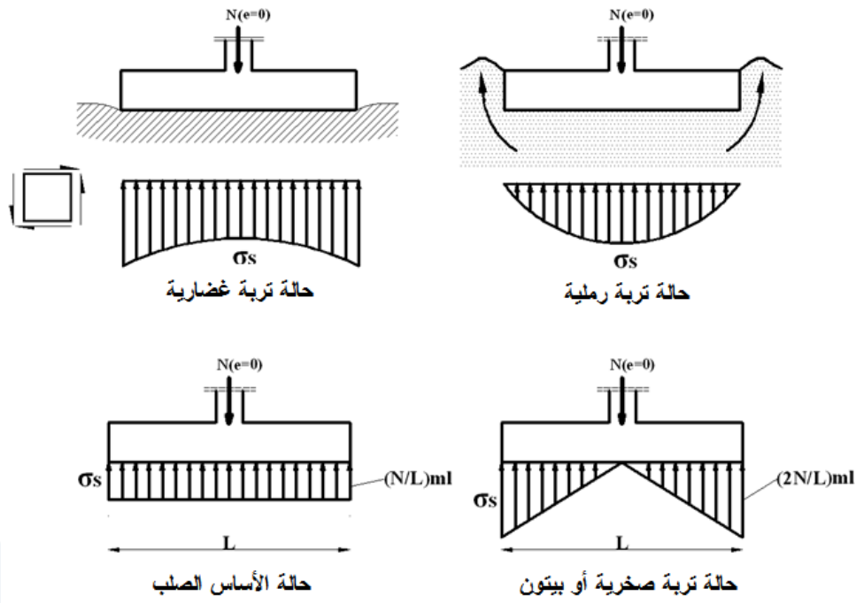
الشكل (5-19): توزيع ضغط التربة تحت الأساس (حمولة مركزية)
