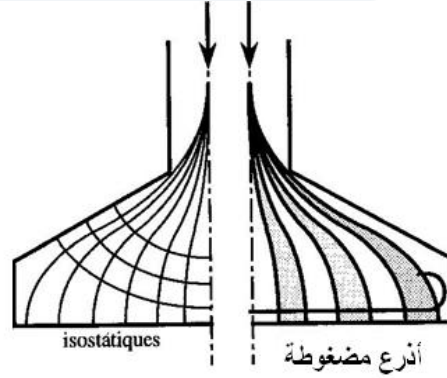
الشكل (5-32): تشكل أذرع الضغط في أساس من البيتون المسلح
