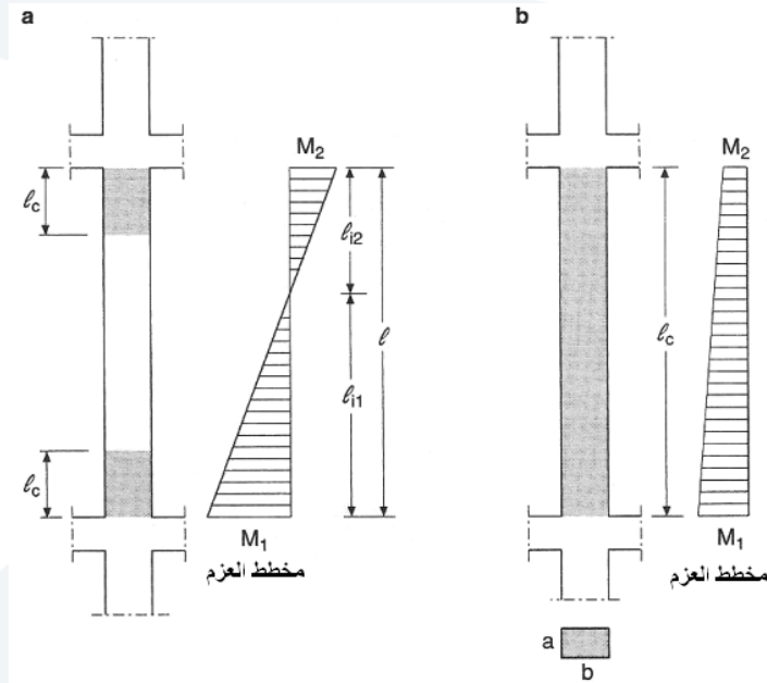
الشكل (5-69): المناطق الحرجة لعمود ما
