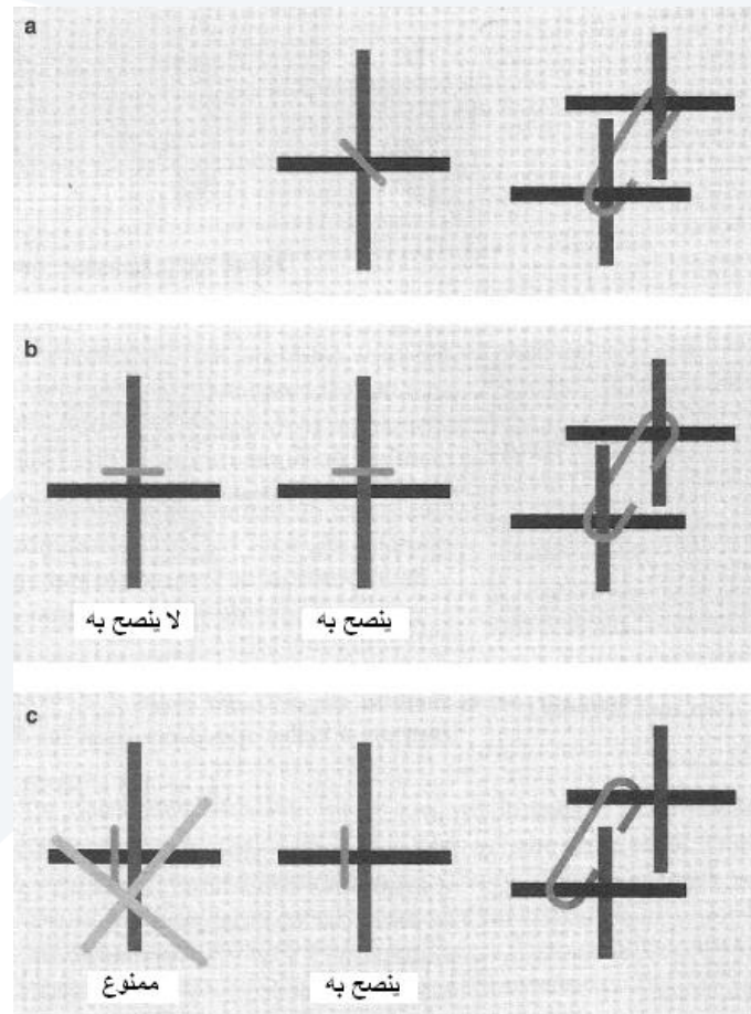
الشكل (5-130): ترتيبات الشناكل (لمنع تحنيد التسليح الشاقولي ونقل الجهود في مناطق التراكب)
