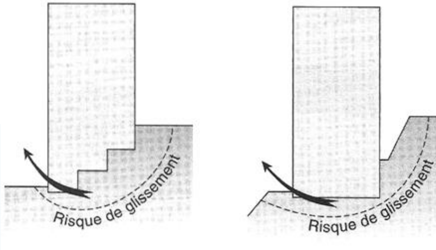
الشكل (3-5): خطر عدم الاستقرار بسبب الانحدار (الانزلاق)
