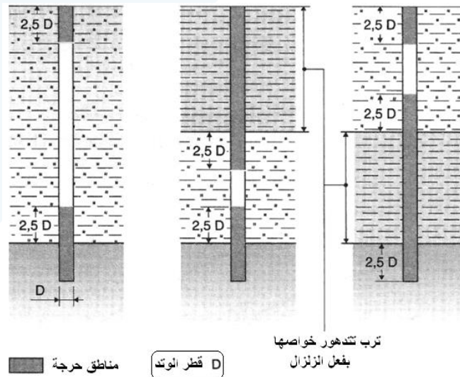
الشكل (5-18): المناطق الحرجة في الأوتاد
