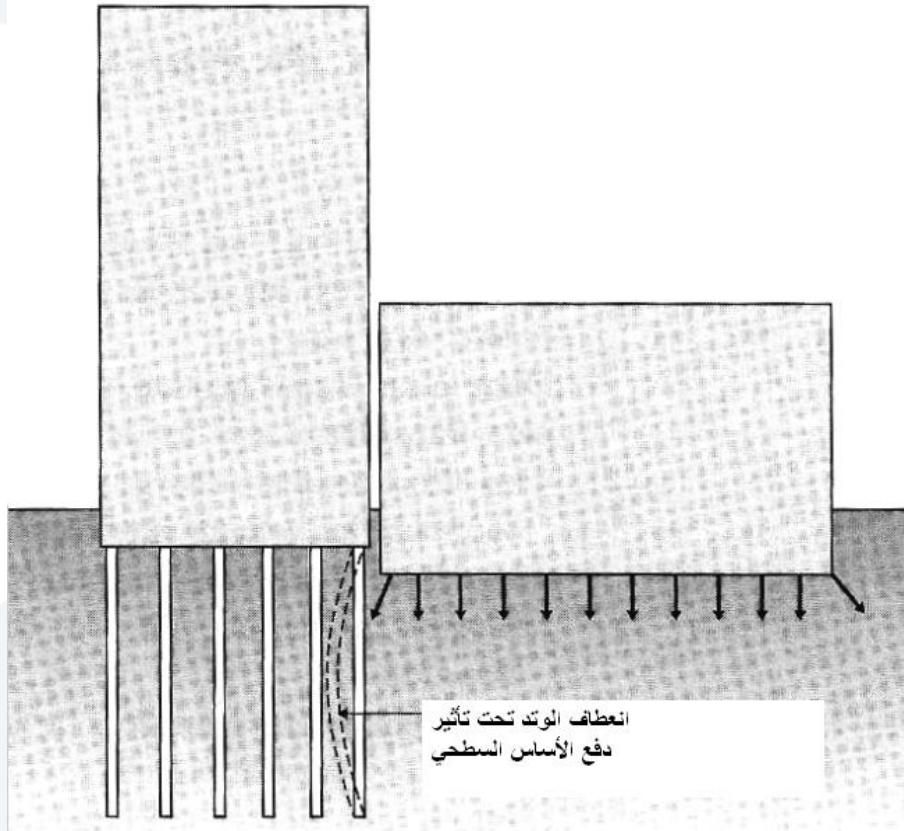
الشكل (2-5): التداخل بين الأساسات السطحية والعميقة
