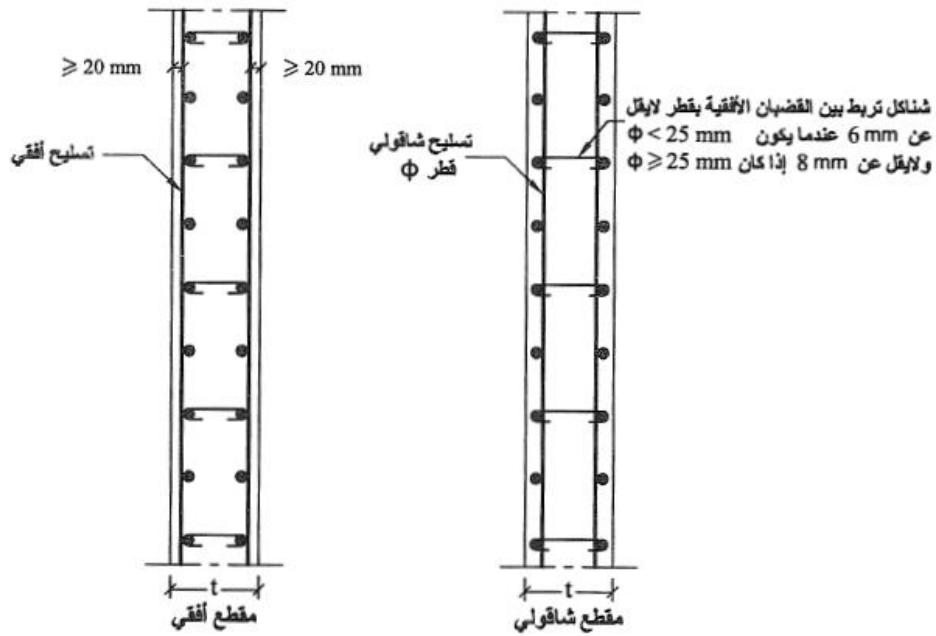
الشكل (5-141): تسليح الجدران الحاملة
