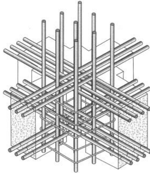
الشكل (5-117): تسليح عقدة وسطية
