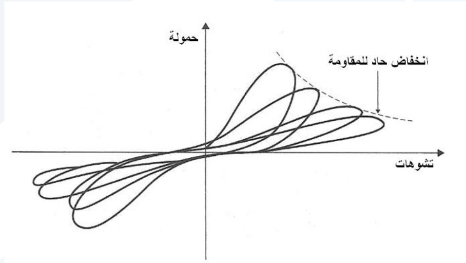
الشكل (5-7): سلوك العناصر الإنشائية تحت تأثير حمولات متناوبة
