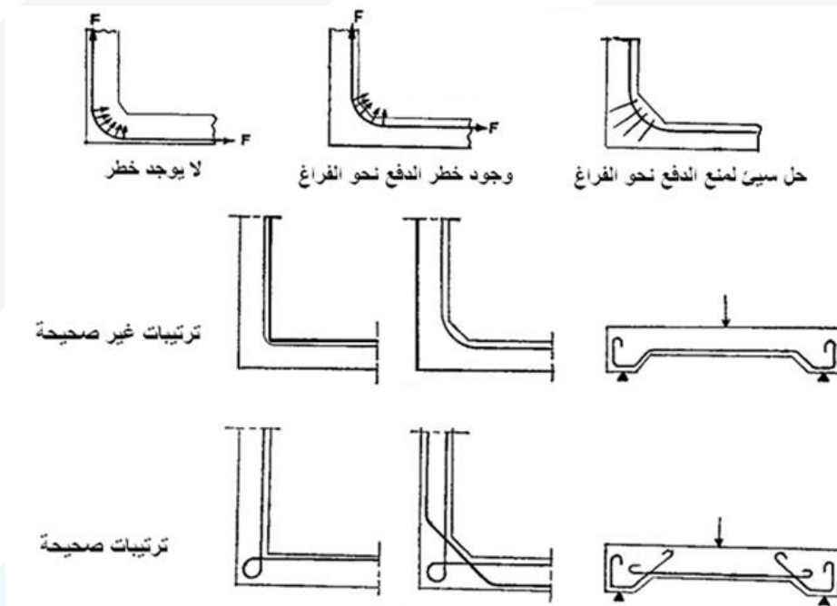
الشكل (5-65): ترتيبات لتجنب قوى الدفع نحو الفراغ عند الزوايا
