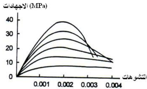
الشكل (46-5): مخطط الإجهادات والتشوهات لعينات نظامية من البيتون، خاضعة لضغط مركزي
