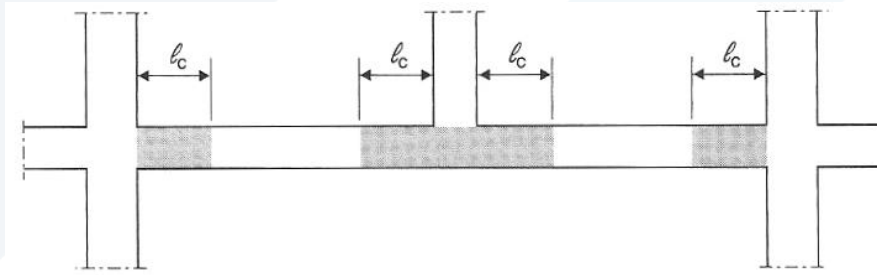
الشكل (5-96): المناطق الحرجة لجوائز حامل لعمود
