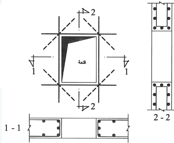
الشكل (5-142): التسليح حول الفتحة في الجدار الحامل
