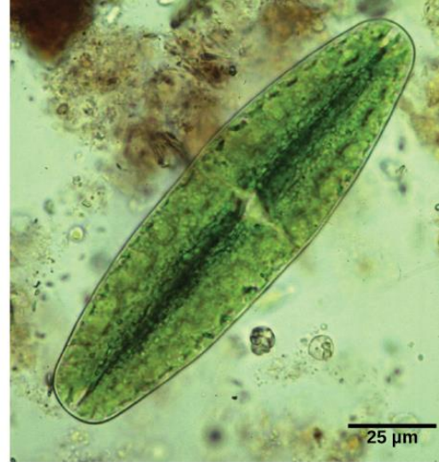
(b) Desmid
