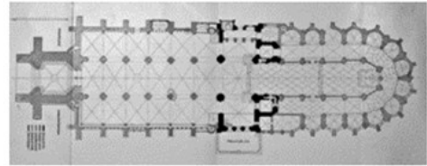
كاتدرائية فرايبورغ: منظور - مسقط - المجاز المركزي - واجهة غربية
