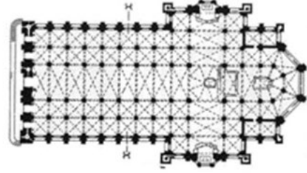
كاتدرائية ميلانو: مقطع عرضي - مقطع طولي - مسقط - واجهة غربية - المجاز المركزي
