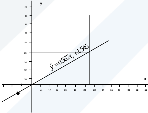
شكل (6-7) يبين مستقيم انحدار y على x (تقريبي)
