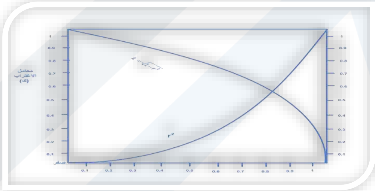
شكل (5-6): العلاقة بين معامل الارتباط r ومعامل التحديد r^2 ومعامل الاغتراب k^2
